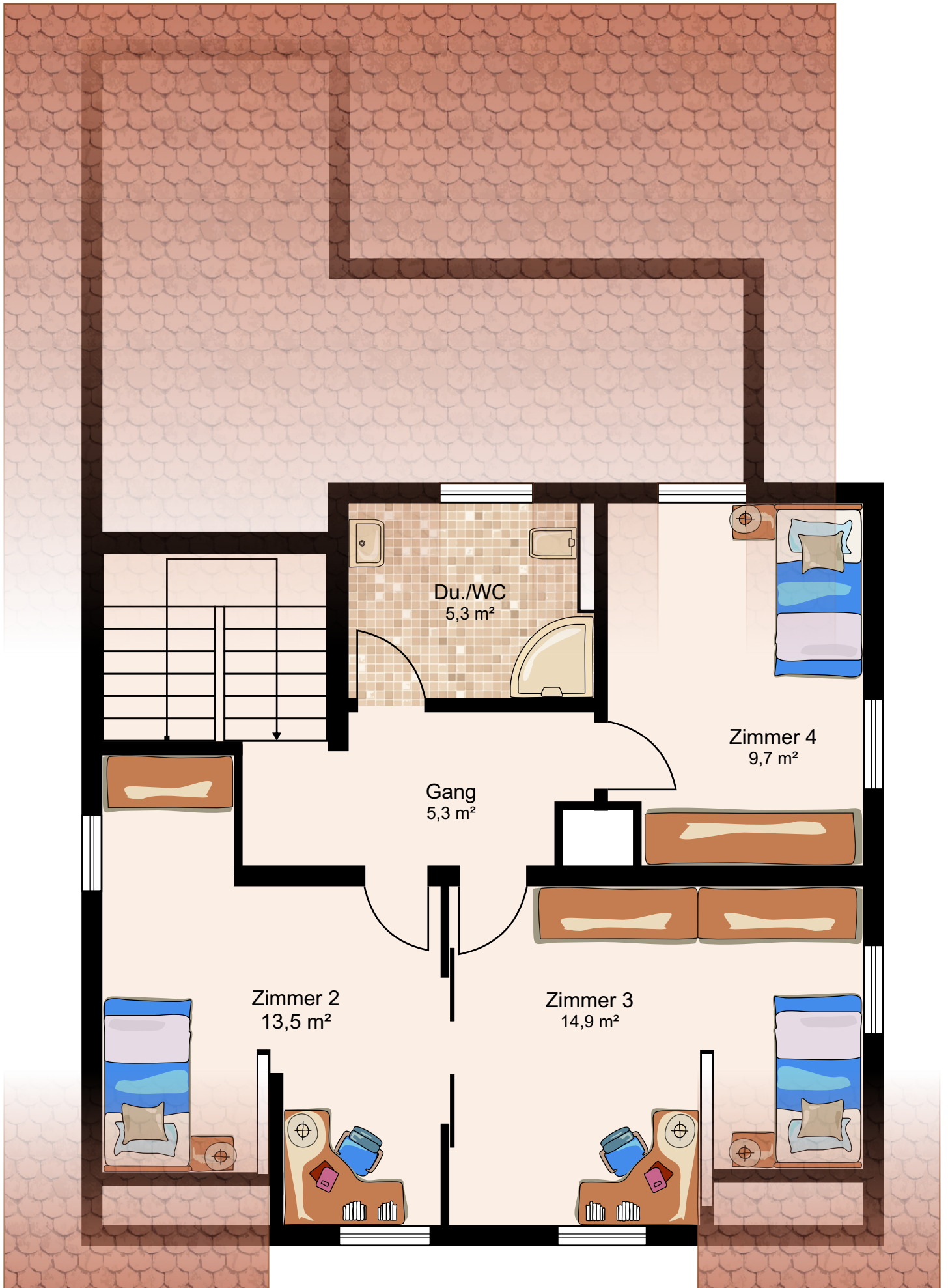
Obergeschoss
